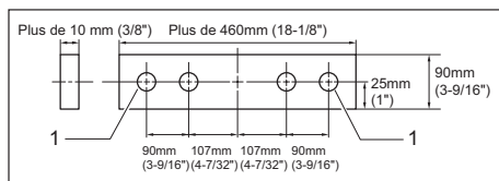
1. Orifice
