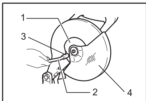
► 1. Cubierta central 2. Llave de tubo 3. Tornillo hexagonal 4. Protector de disco
