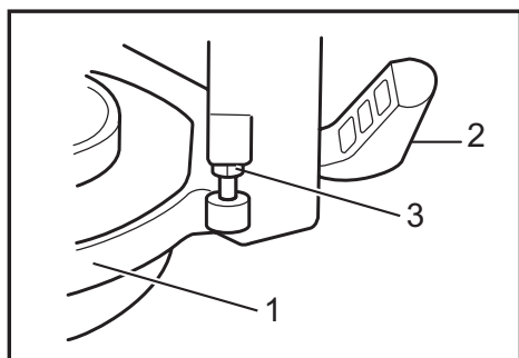
► 1. Base giratoria 2. Palanca 3. Tornillo de ajuste a 0°
