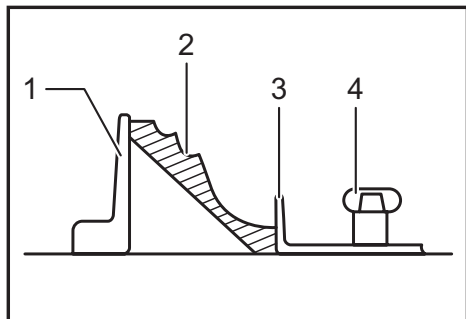
► 1. Garde de guidage 2. Moulure couronnée 3. Butée de moulure couronnée 4. Vis
