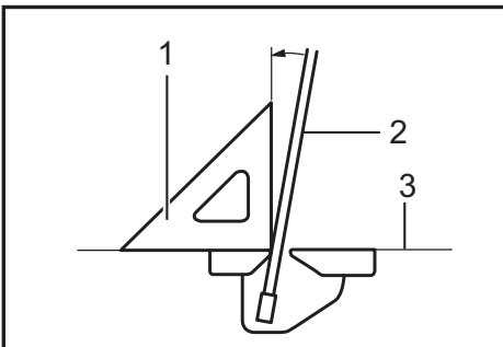
► 1. Règle triangulaire 2. Lame 3. Face supérieure du
