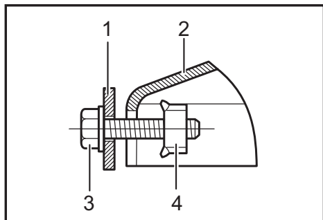
► 1. Auxiliary plate 2. Base 3. Hex bolt 4. Nut
