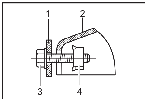
► 1. Plaque auxiliaire 2. Base 3. Boulon hexagonal 4. Écrou
