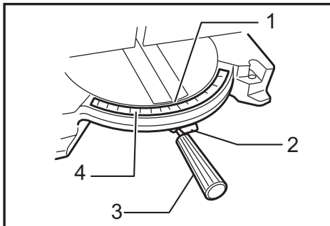
► 1. Puntero 2. Palanca de bloqueo 3. Empuñadura 4. Escala de inglete
