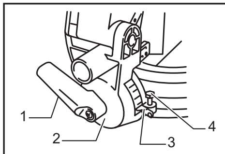
► 1. Palanca 2. Brazo 3. Puntero 4. Ángulo bisel de 45° mediante el ajuste del tornillo
