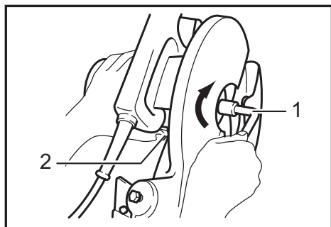
► 1. Llave de tubo 2. Bloqueo del eje
