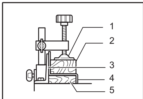
► 1. Étau 2. Cale d'espacement 3. Garde de guidage 4. Profilé d'aluminium 5. Cale d'espacement
